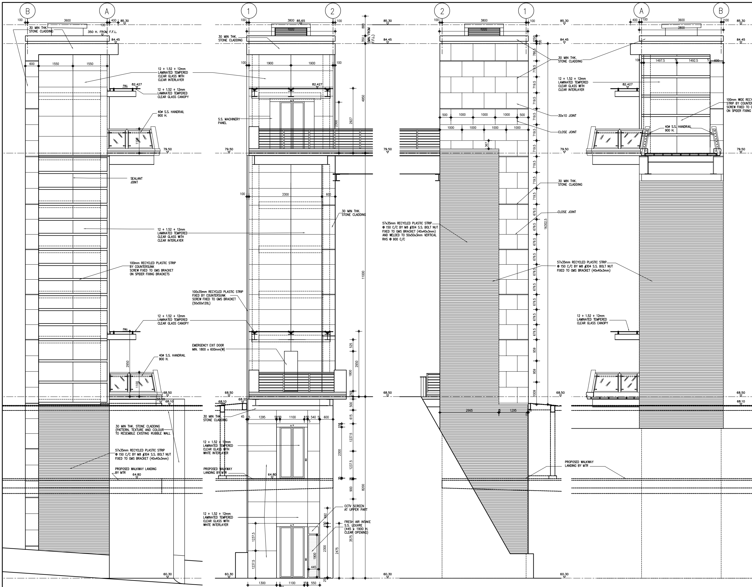
ELEVATION A
